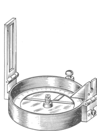
Рис. 112. Ручная буссоль Шмалькальдера
