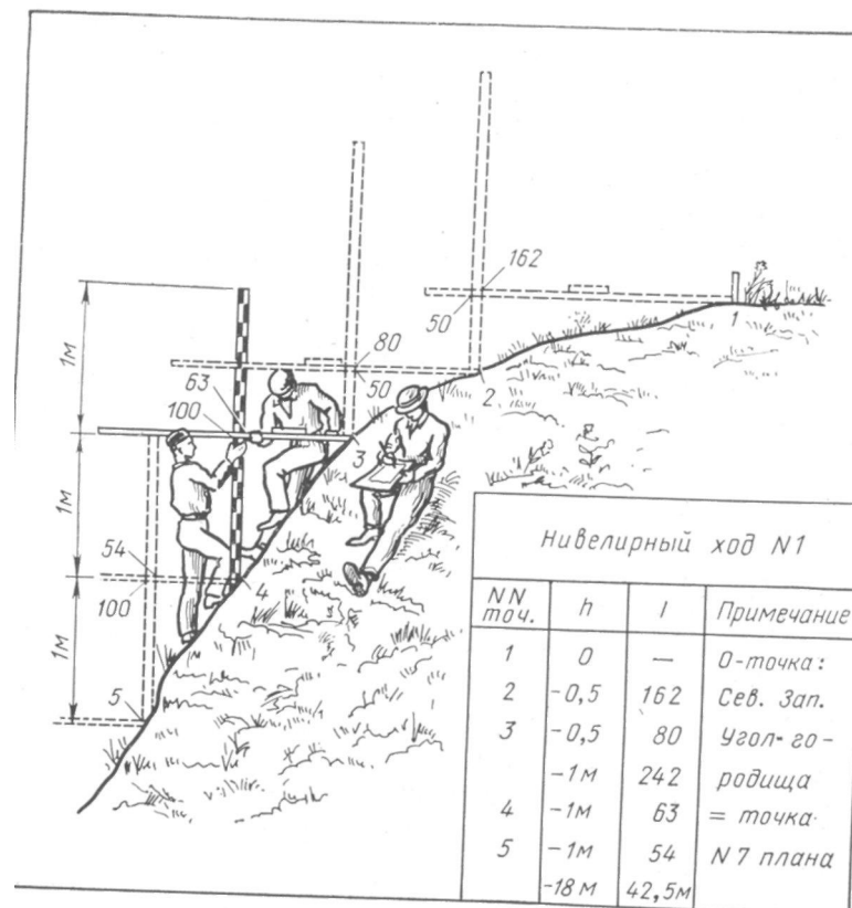
Рис. 123. Нивелирование скатов с помощью реки и уровня
