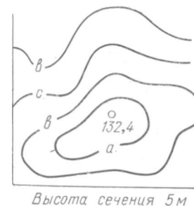
Рис. 103. Определение отметки горизонтали по отметке точки:
