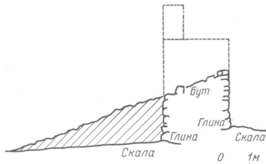
Рис. 66. Опыт восстановления высоты стены Харакса по ее завалу. (По В. Д. Блаватскому)
