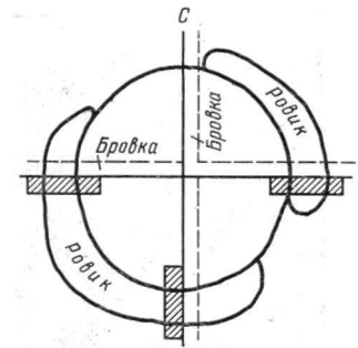
Рис! 42. План траншеек для исследования насыпи и ровиков:
