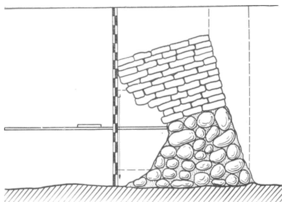
Рис. 92. Промеры через нависший край
