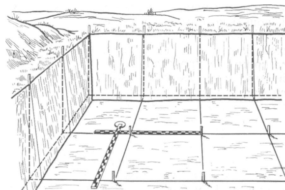
Рис. 76. Правильный замер координат (от угловых кольев квадрата)
