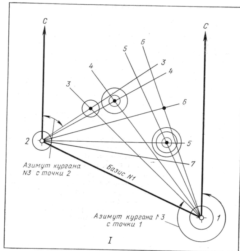
Рис. 120. Съемка плана способом засечек. (По М. Н. Кислову)
