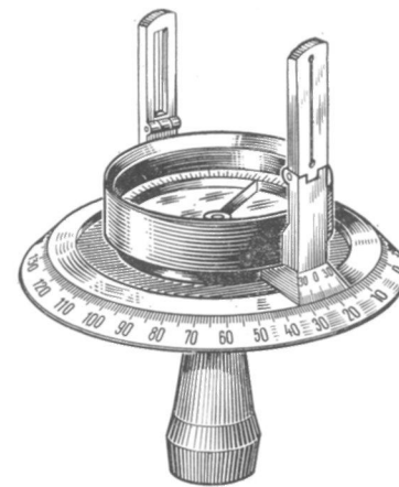
Рис. 113. Штафивная буссоль Стефана
