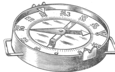
Рис. ПО. Компас Адрианова
